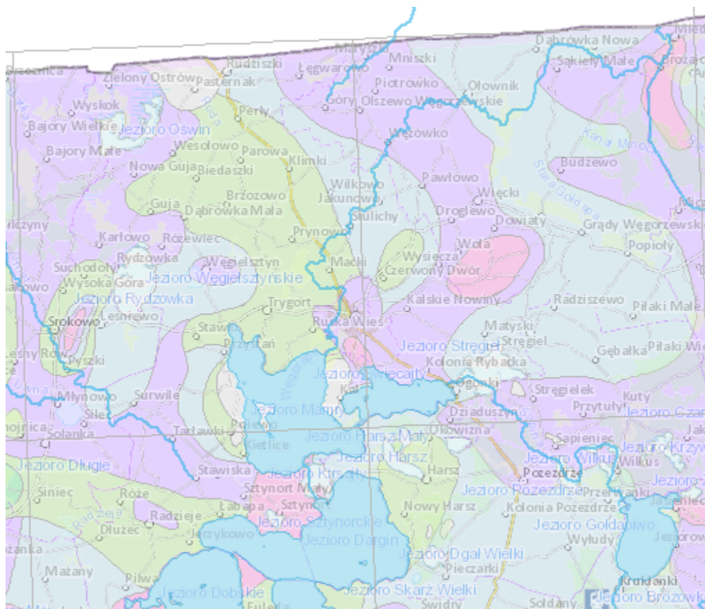
Rysunek 3 Wydajność potencjalna studni na terenie powiatu węgorzewskiego
